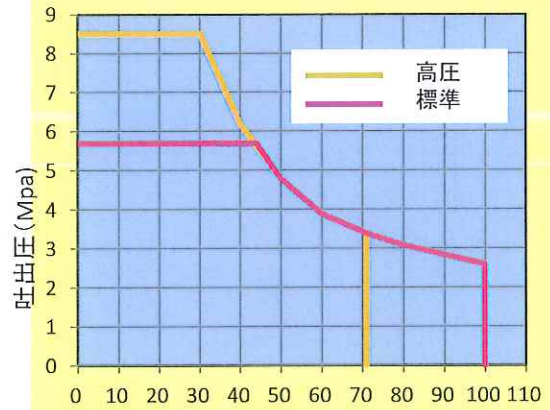
BSF20.09H ホンプ能力線図(理論図)
